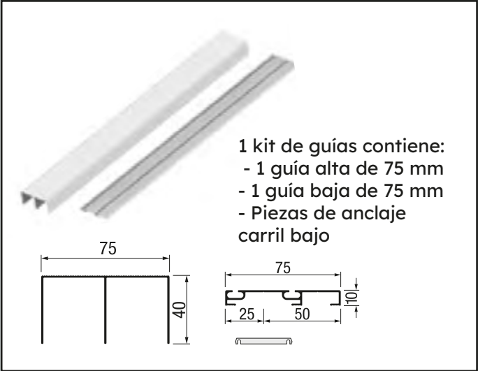
Kit guías 16 mm carril de 75 mm
