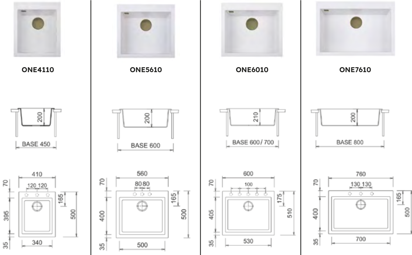
Medidas mecanizado según modo de instalación
