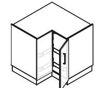
LBR2D Derecha A 93 x 93 P 60 H 80
