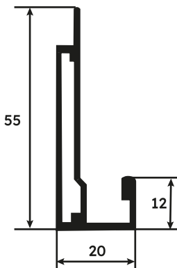
Perfil para tablero de 10mm
