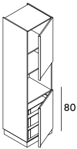
ACH2 A 60 P 60 H 220/230
